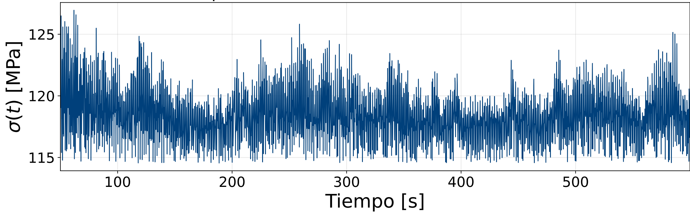
Serie temporal de tensión en la sección crítica ( V = 10 m/s)
